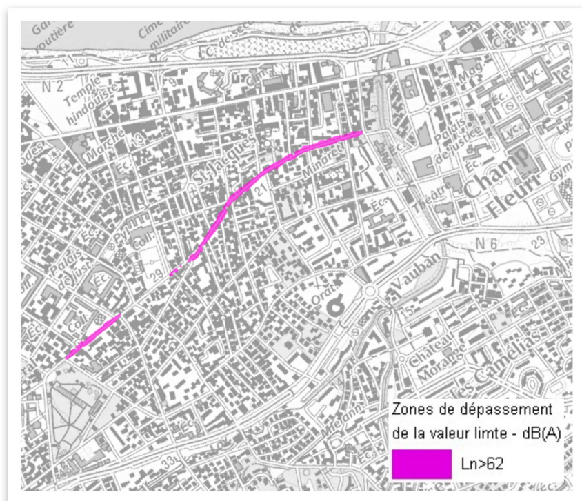
Figure 12 : Exemple de cartographie de type C L_n - rue du Maréchal Leclerc - commune de Saint Denis
